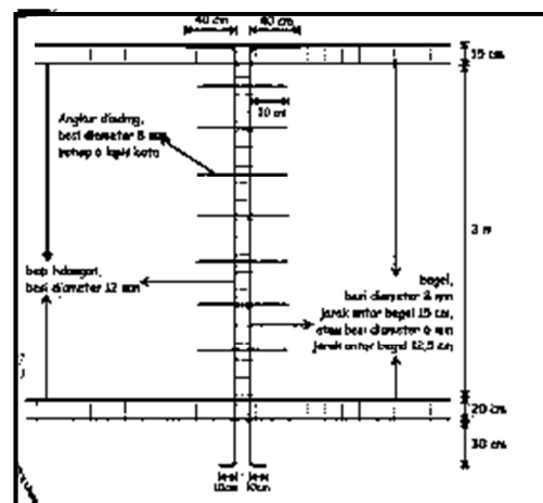
Gambar 11. Detail Pengangkuran Kolom pada Dinding (Sumber ; Hasil Analisis)
