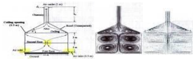
Gambar 6. Model Fisik bangunan, pola streamline dan pola Velocity vectors (Chitsomboon, 2004)
