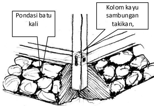
Gambar 3.12. Tipe pondasi rumah bajo tipe 3.
