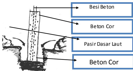
Gambar 9. Tiang Rumah Suku Bajo Tipe 2
