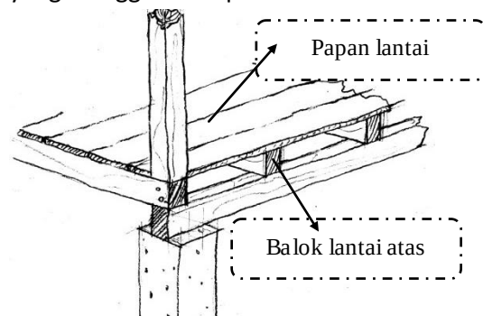
Gambar 10. konstruksi dinding rumah suku Bajo tipe 2.
